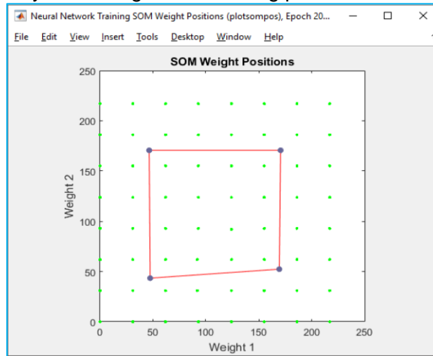
Figure 7: SOM Weight Positions
